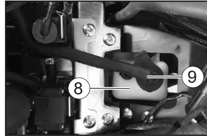
8. Kühlmittel flüssigkeit tank 9. Deckel des Kühlmittel tanks
