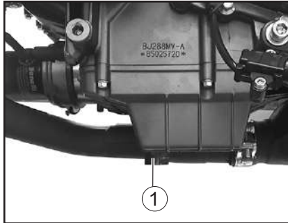
1. Motoröl-Ablassschraube
